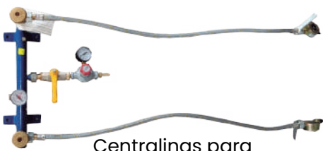
Centralinas para 2 cilindros de gas
