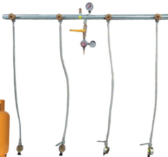
Centralinas para 4 cilindros de gas
